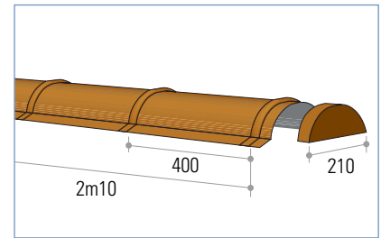
9 faîtière et embout de faîtière
